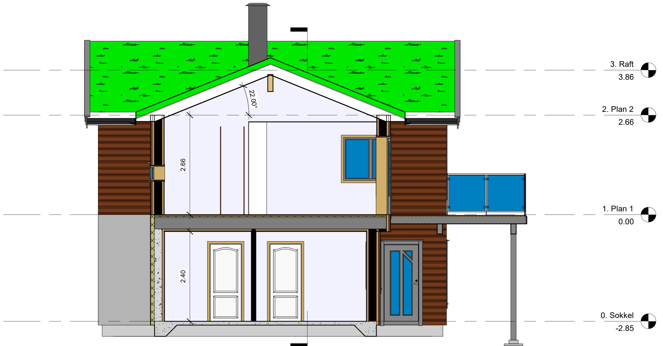
1 Section YY 1 : 50
