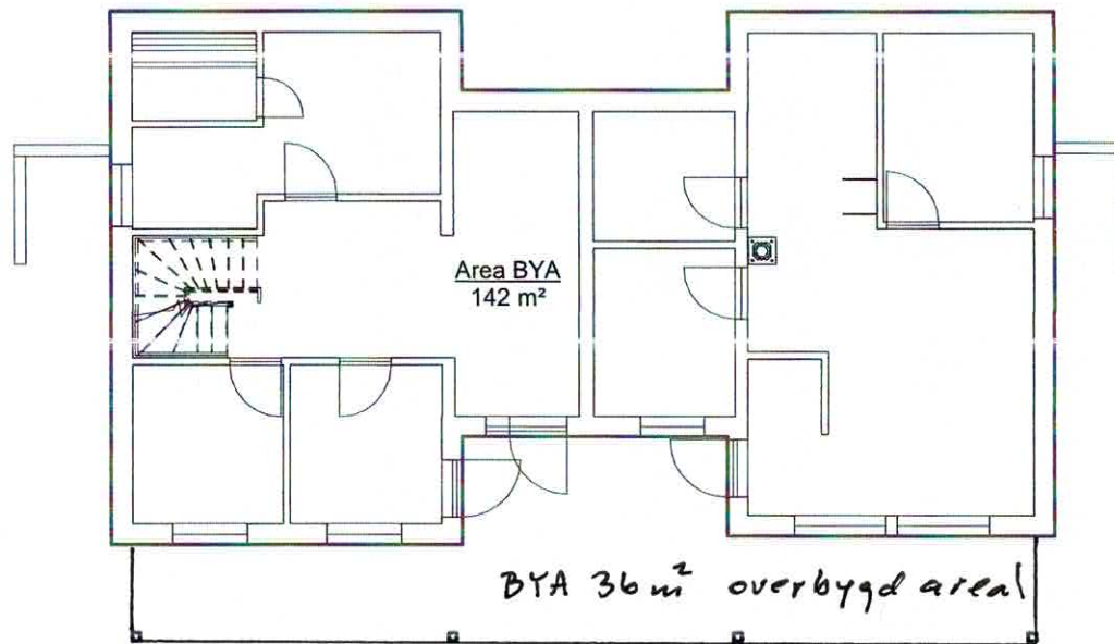
1 0. Sokkel 1 : 100
