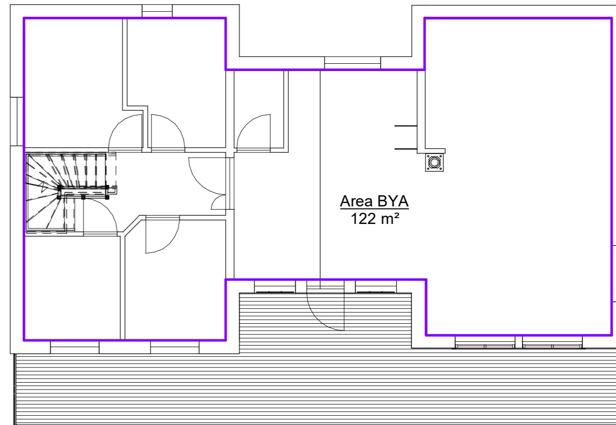
2 1. Plan 1 1 : 100
