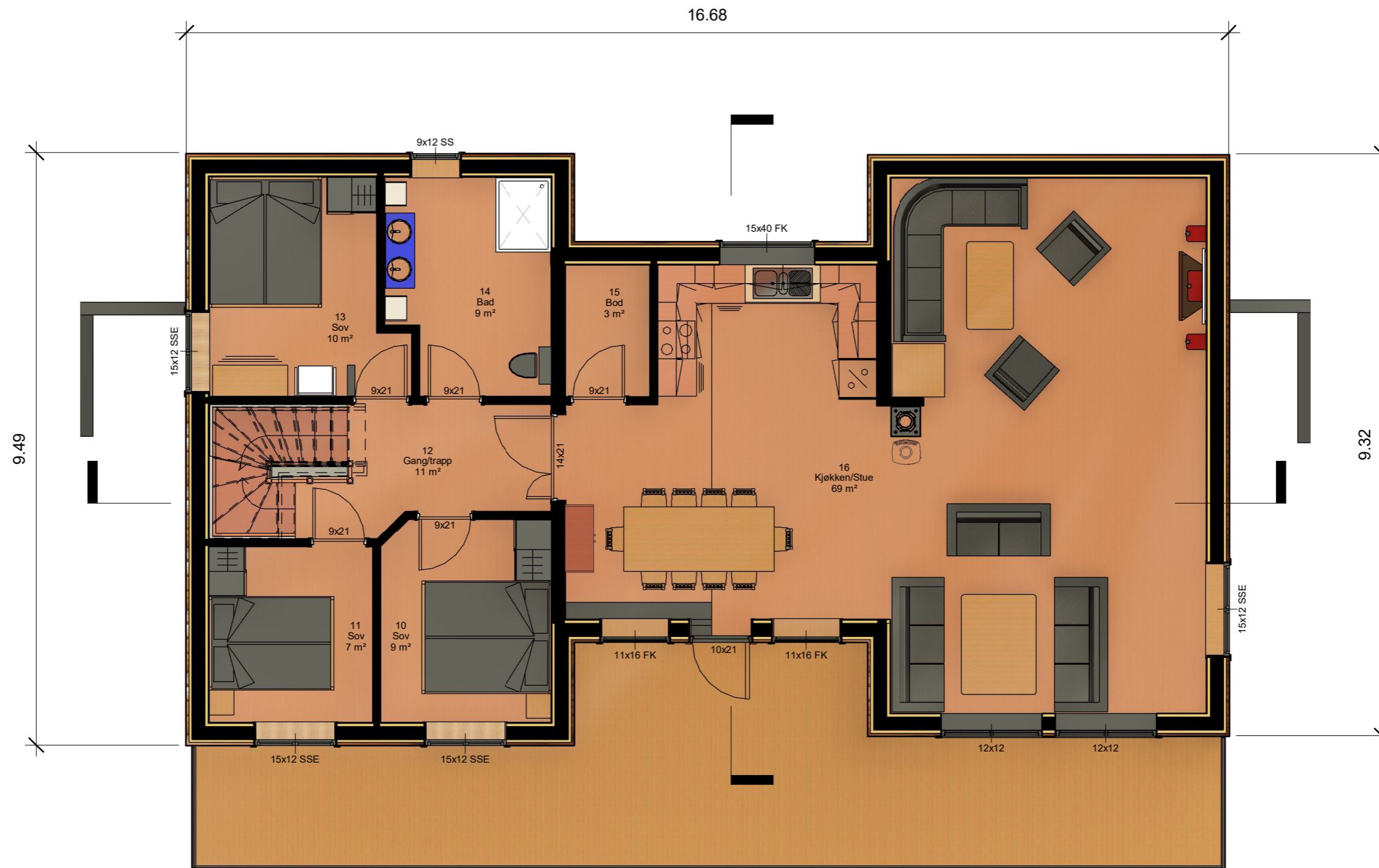
1 1. Plan 1 1 : 75
